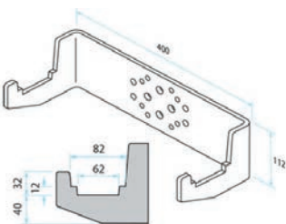
Inox Haken 60 - 80 mm Artikel Nr 335872
