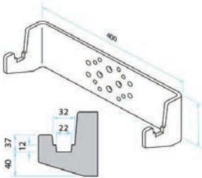
Inox Haken 20 - 30 mm Artikel Nr 336485
