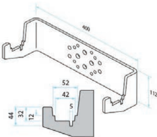
Inox Haken 5 - 40 - 50 mm Artikel Nr 335865
